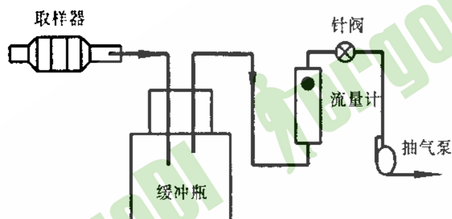
图 1 空气采样系统组成示意图
