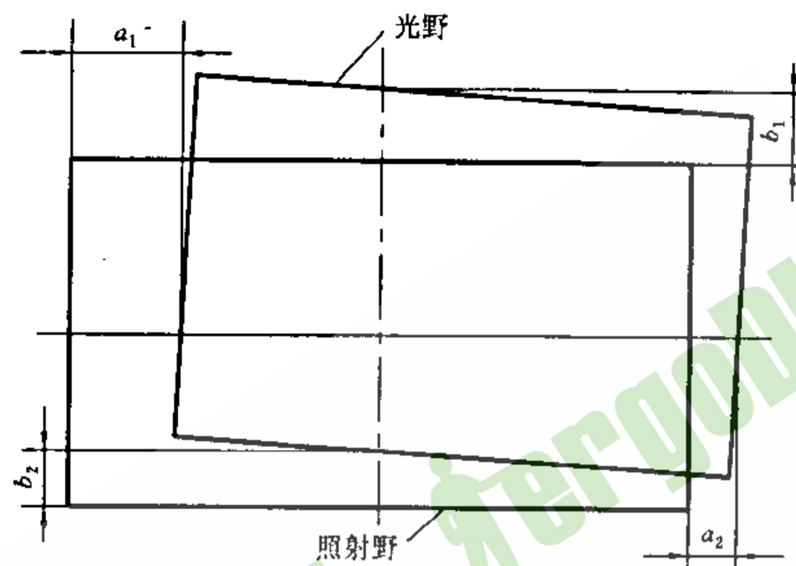
图 C3 光野与照射野的偏离
