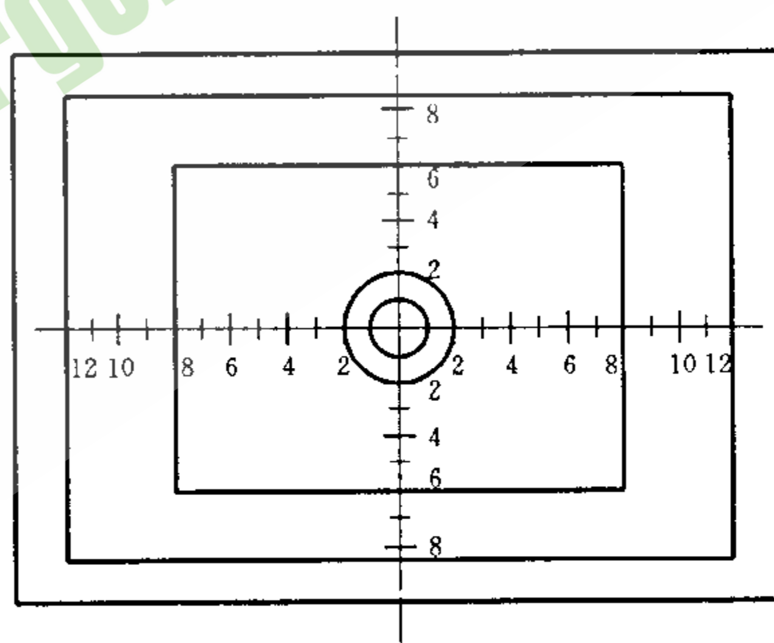
图 C2 准直测试板
