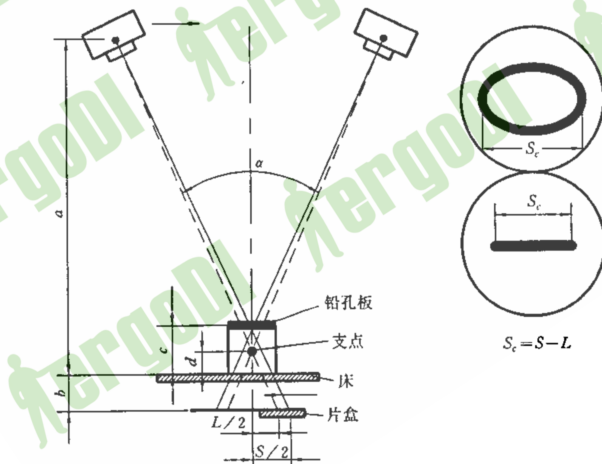
图 E1 断层扫描曝光角度检测方法示意图
