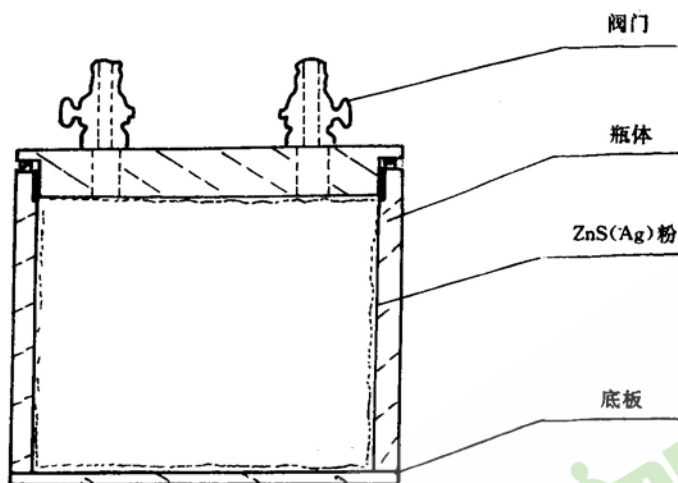
图1 闪烁瓶简图
